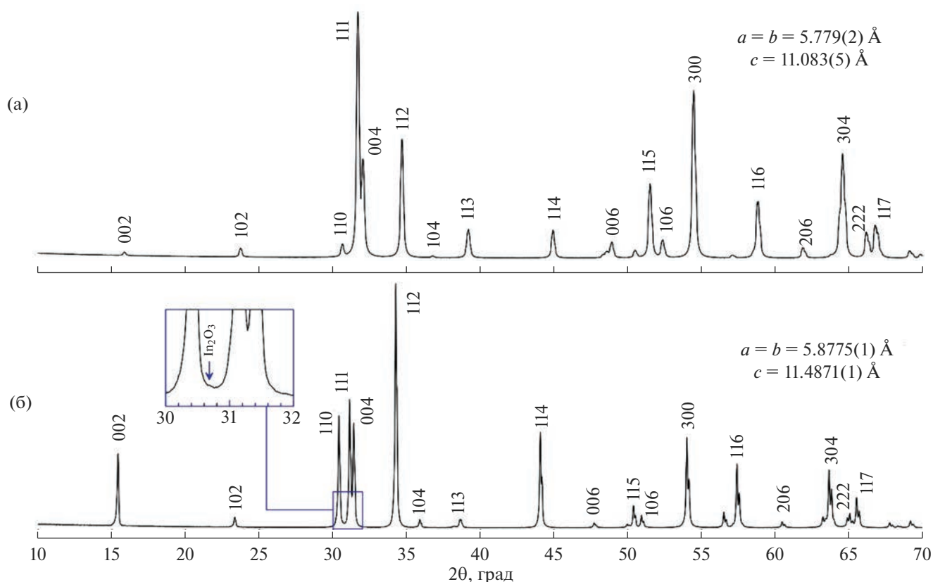
Рис. 3. Рентгенограммы манганитов \text{ScMn}_{0.996}^{57}\text{Fe}_{0.004}\text{O}_3 (а) и \text{In}_{0.97}(\text{Mn}_{0.99}^{57}\text{Fe}_{0.01})_{1.03}\text{O}_3 (б). Указанные индексы рефлексов hkl соответствуют пр. гр. P6_3cm . На вставке к панели (б) изображен фрагмент рентгенограммы с рефлексом 222 примесной фазы \text{In}_2\text{O}_3 .
