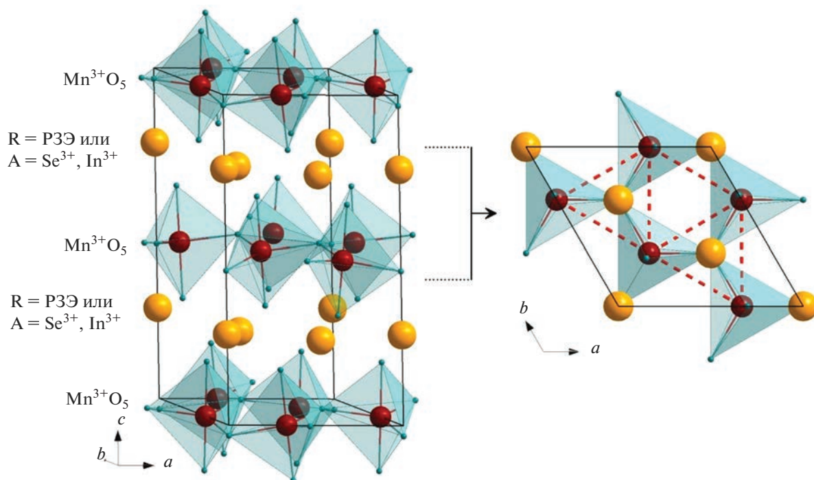
Рис. 1. Фрагмент кристаллической структуры манганитов h\text{-AMnO}_3 (пр. гр. P6_3cm ) в разных проекциях.
