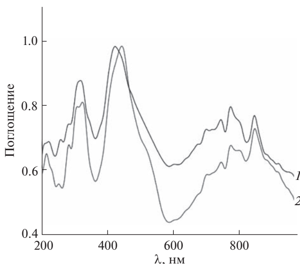
Рис. 4. Спектры образцов \text{Mg}_{3-n}\text{Ni}_n\text{BPO}_7 : n = 3 (1) и 1.5 (2) в УФ-видимом и ближнем ИК-диапазоне.
